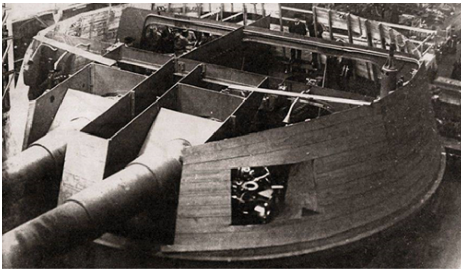
Бронешашенная бататрея-30 на этапе строительства
